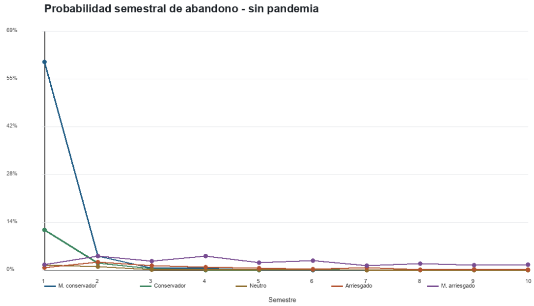
Figura 3: Probabilidad semestral de abandono sin pandemia para Momentum general con abandono V1.
