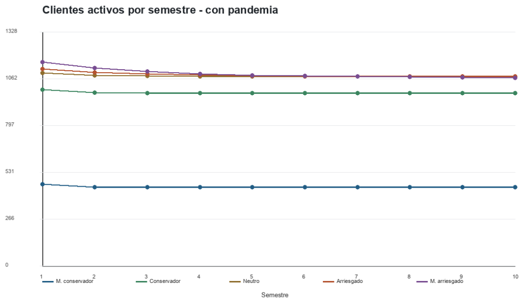
Figura 2: Clientes activos por semestre con pandemia para Momentum general con abandono V1.
