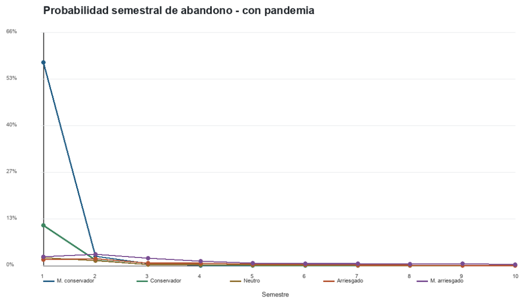
Figura 4: Probabilidad semestral de abandono con pandemia para Momentum general con abandono V1.
