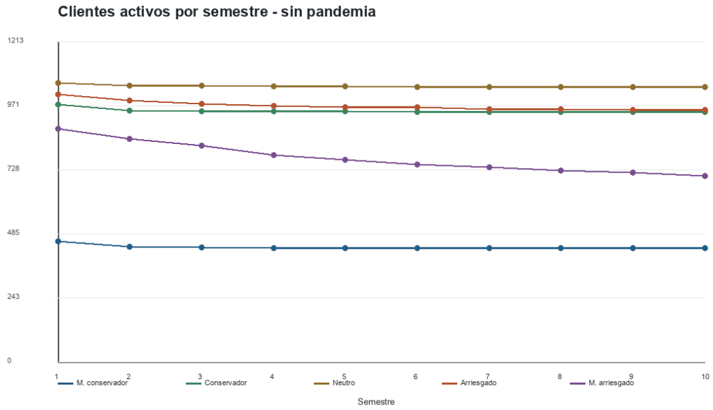
Figura 1: Clientes activos por semestre sin pandemia para Momentum general con abandono V1.
