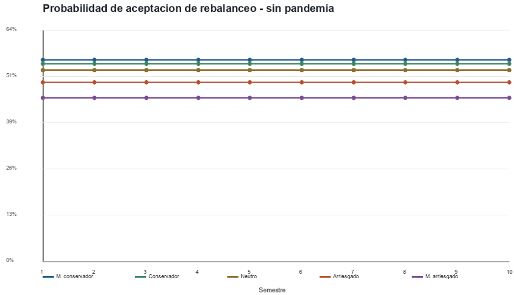
Figura 5: Probabilidad semestral de aceptación de rebalanceo sin pandemia para Momentum general con abandono V1.
