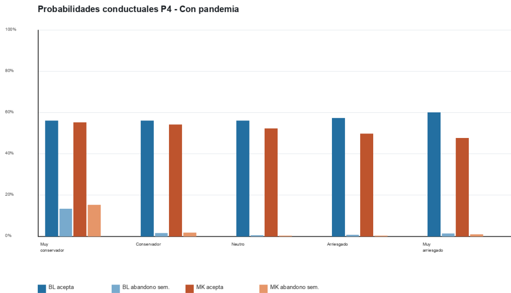
Figura 8: Probabilidades conductuales con pandemia para Momentum general con abandono V1.
