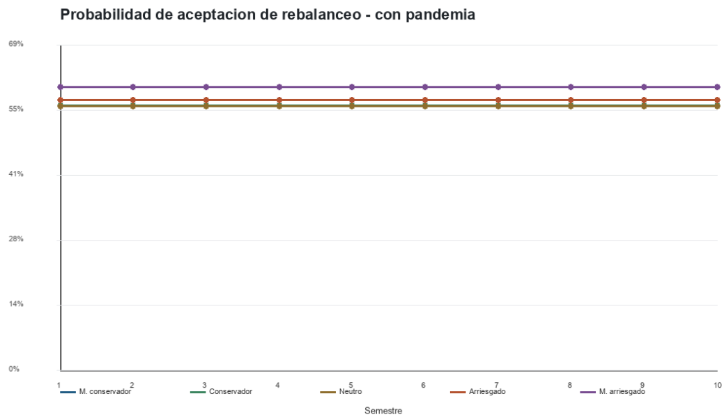
Figura 6: Probabilidad semestral de aceptación de rebalanceo con pandemia para Momentum general con abandono V1.
