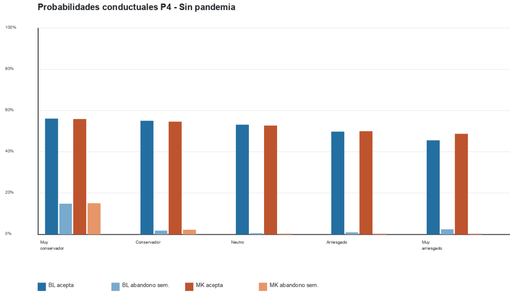
Figura 7: Probabilidades conductuales sin pandemia para Momentum general con abandono V1.
